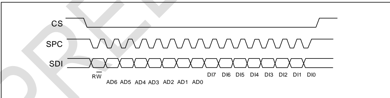
SPI写协议
